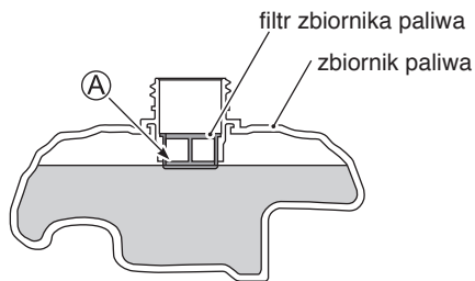
Ⓐ: Filtr siatkowy na spodzie filtra
