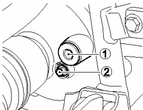
Przedni dyferencjał
