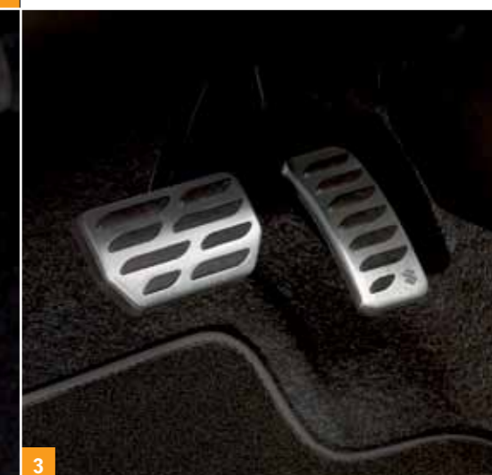
3 | Sportowe nakładki pedałów aluminiowe, do wersji z kierownicą po lewej stronie do wersji z manualną skrzynią biegów (brak ilustr.) Nr ewid. 990E0-61M93-000 do wersji z automatyczną skrzy- nią biegów Nr ewid. 990E0-61M93-001
